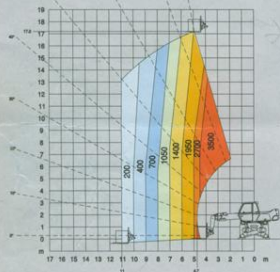
ROTAZIONE SU STABILIZZATORI PARZIALMENTE SFILATI CON FORCHE
